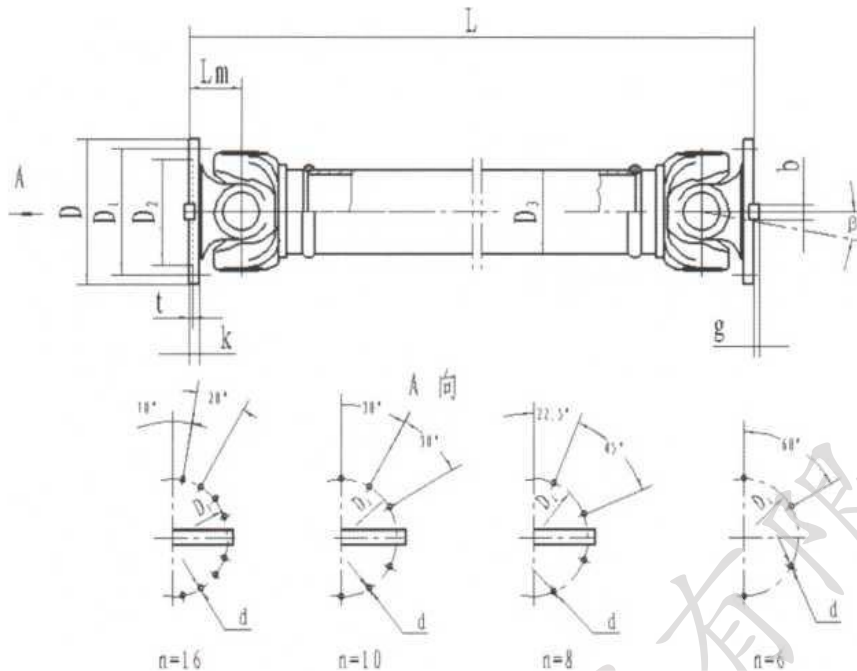
SWC WH 型（无伸缩焊接型） 整体叉头十字轴式万向联轴器基本参数和主要尺寸（JB/T 5513-1991）
